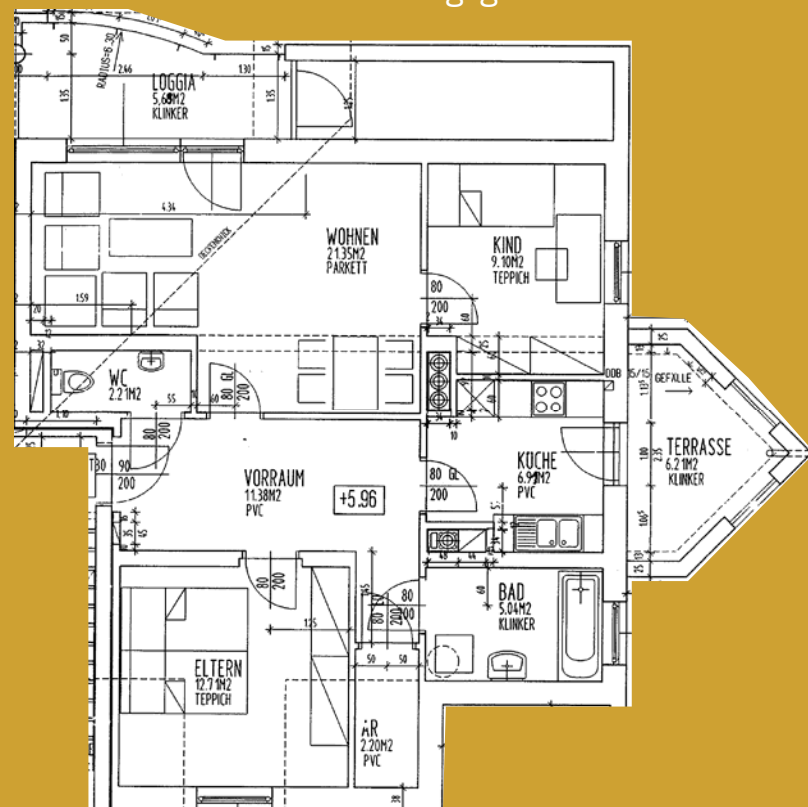
Wohnungsgrundriss
